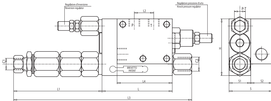
SCHEMA DI MONTAGGIO MOUNTING DIAGRAM
